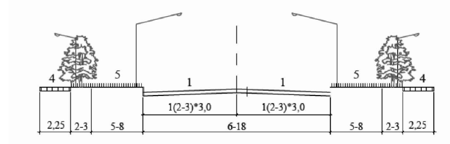
Поперечний профіль дороги районного значення
